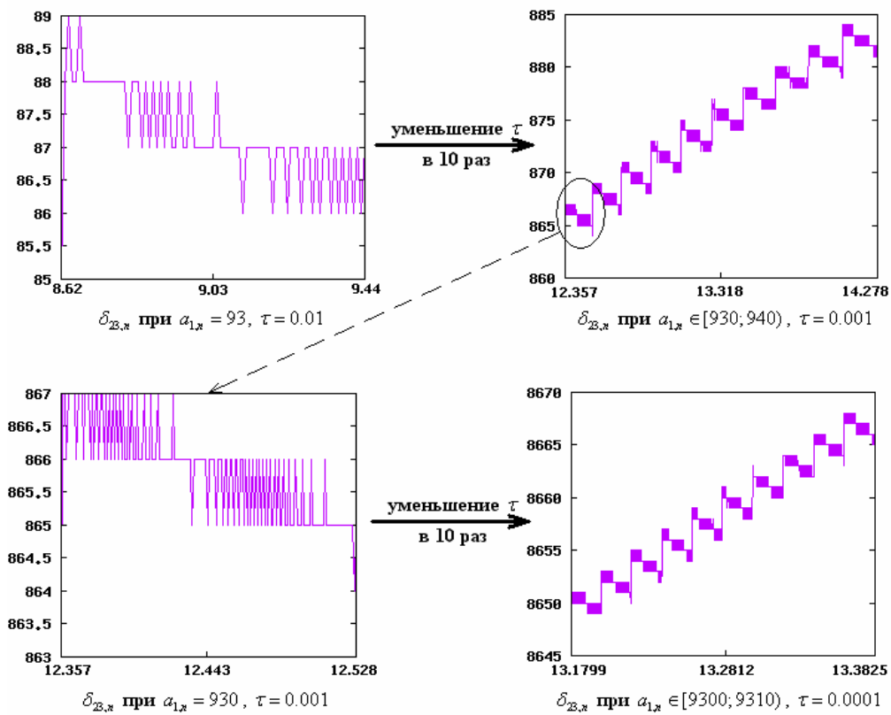
Рис. 3. Применение последовательного «увеличения» (т.е. уменьшения \tau при фиксированном слое по a_{1,n} ) к функции переброса \delta_{23,n}
