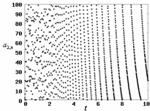
Рис. 1. Зависимость a_{2,n} от t ( A=1 )
