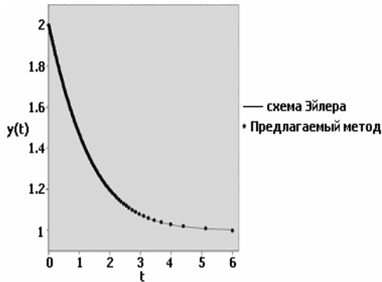
Рис. 4. Решения уравнения (6)
