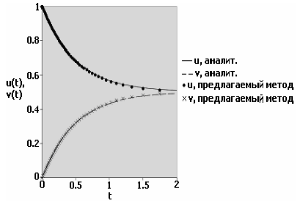
Рис. 5. Решения системы (9)
