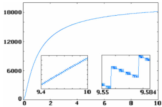
Рис. 2. Зависимость \delta_{23,n} от t ( A=15 )
